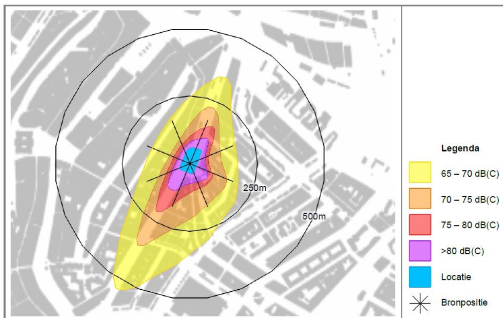
Figuur 3.3.5 Geluidcontouren bij een maximale invulling
